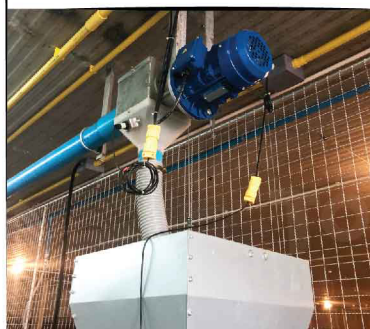
CONTROL PAN ชุดมอเตอร์เกียร์
